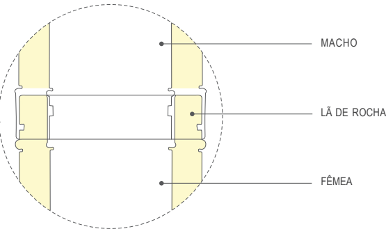
PORMENOR DE ENCAIXE
