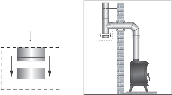
EXEMPLO DE APLICAÇÃO DE TÊ 90° COM TAMPO
